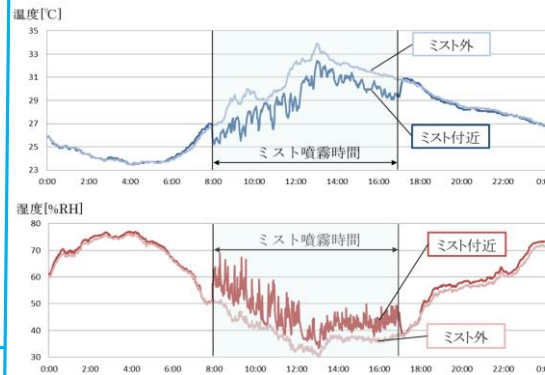
代表点における温湿度推移(2015)
