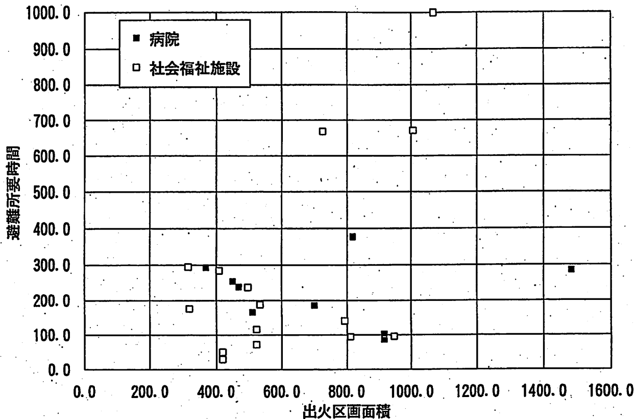
図 2.6: 避難所要時間と出火区画面積 (施設別)
