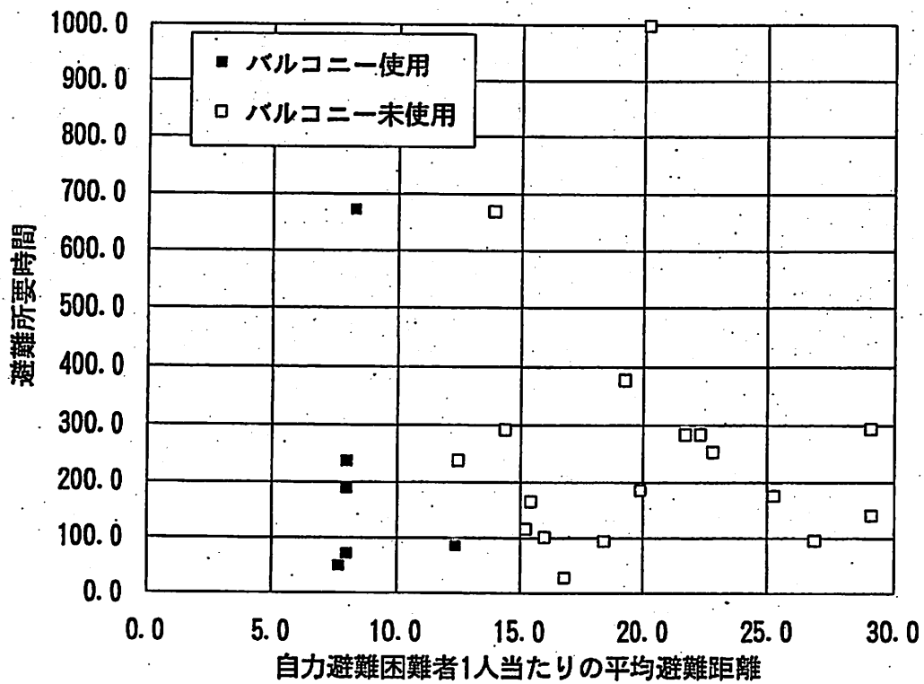
図 2.11: 避難所要時間と平均避難距離 (バルコニー避難の有無)
